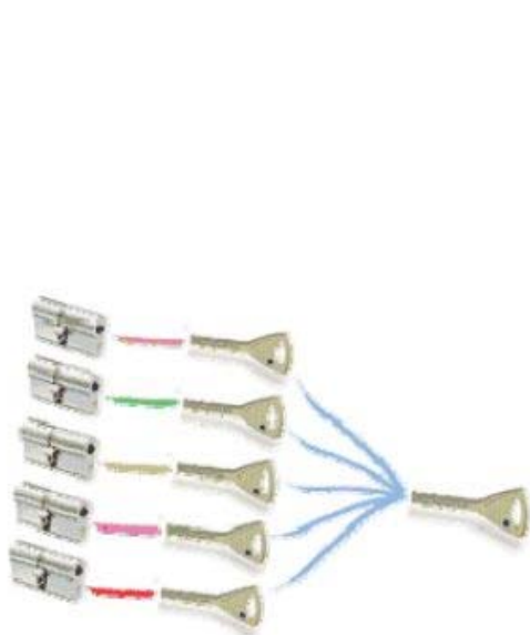
Peavõtme lukustus – Iga võti avab vaid ühe luku, peavõti avab kõik sarja lukud.
