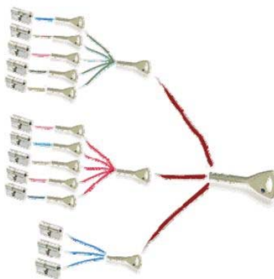
Üldvõtme lukustus – üks ühine peavõti avab kõik lukusüsteemi koondatud lukusüdamikud. Sari koosneb mitmest erinevast lukustuse kombinatsioonist.
