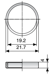
Korotusholkki 804252 - 4 mm (kromattu teräs)
