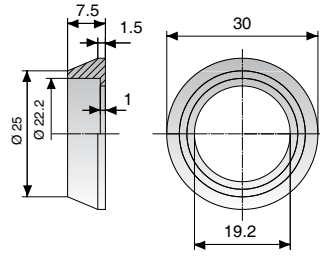
Suojarengas 804757 (kromattu teräs)
