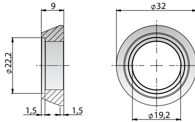
Korotusrengas 812760 - 7,5 mm (kromattu teräs)
