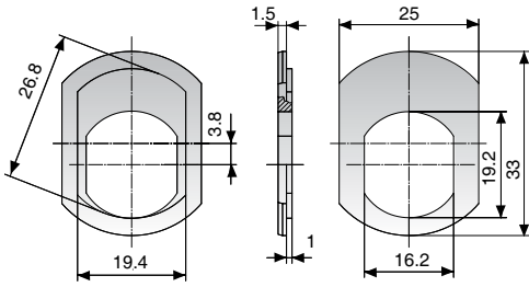
Kiinnityslevy 441345 (kromattu messinki)
