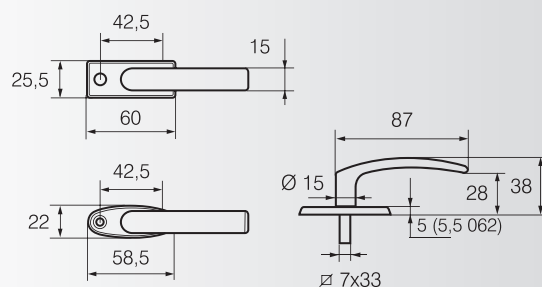
Sinkkipainike
