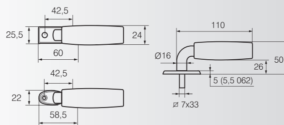
Messinki/lehtikuusi -painike
